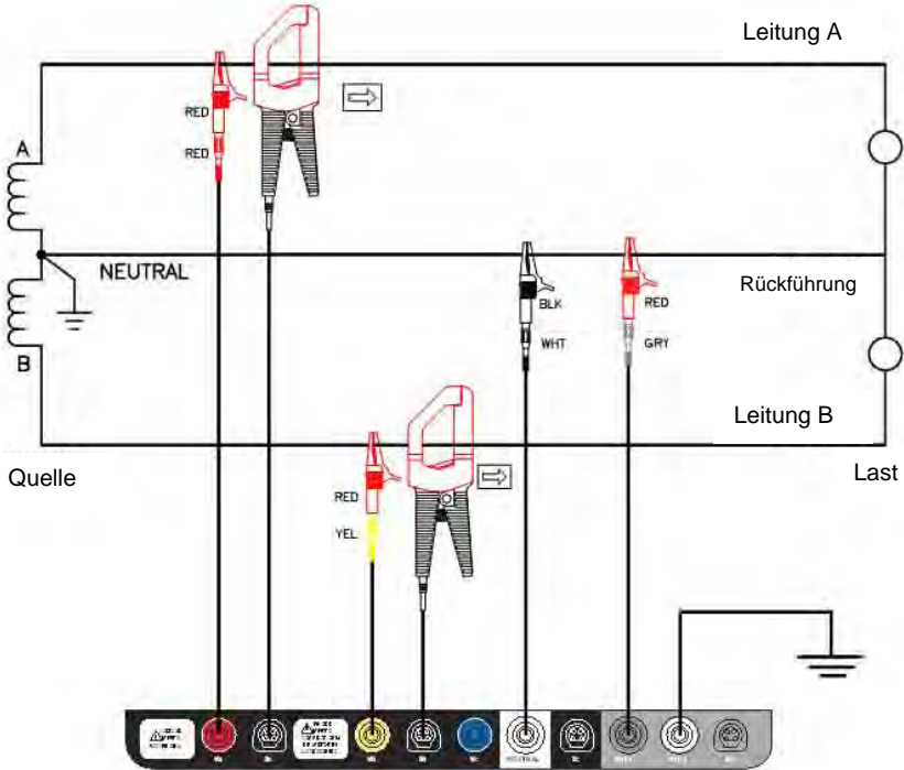
Anschluss Schaltbild
