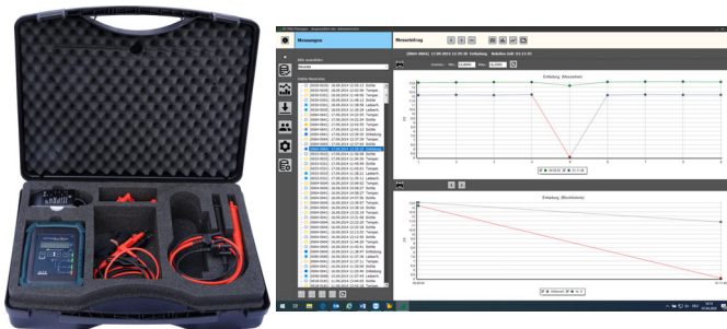
Bild 1: Transportkoffer (links), Messdatenauswertung (rechts)
