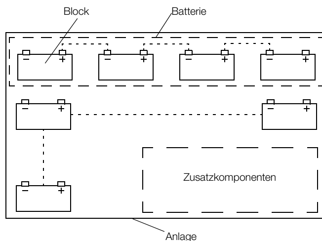
Bild 2: Beispiel - Block und Batterie einer Anlage
